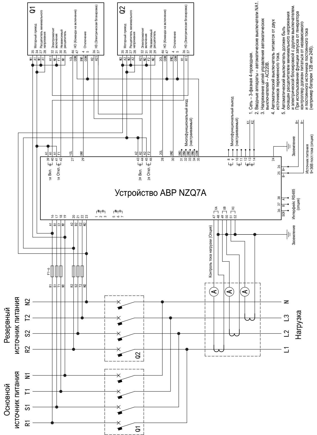
Принципиальная электрическая схема 1 для 3-фазной 4-проводной сети
